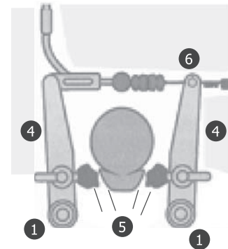
V Brake
